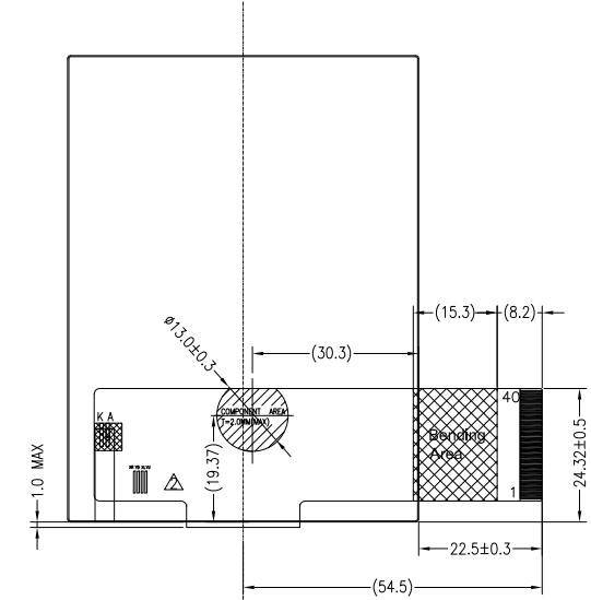
弯折示意图 FPC展开出货
